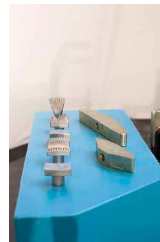
Différents mors de redressage sont fournis, permettant de redresser toute partie de jante.
